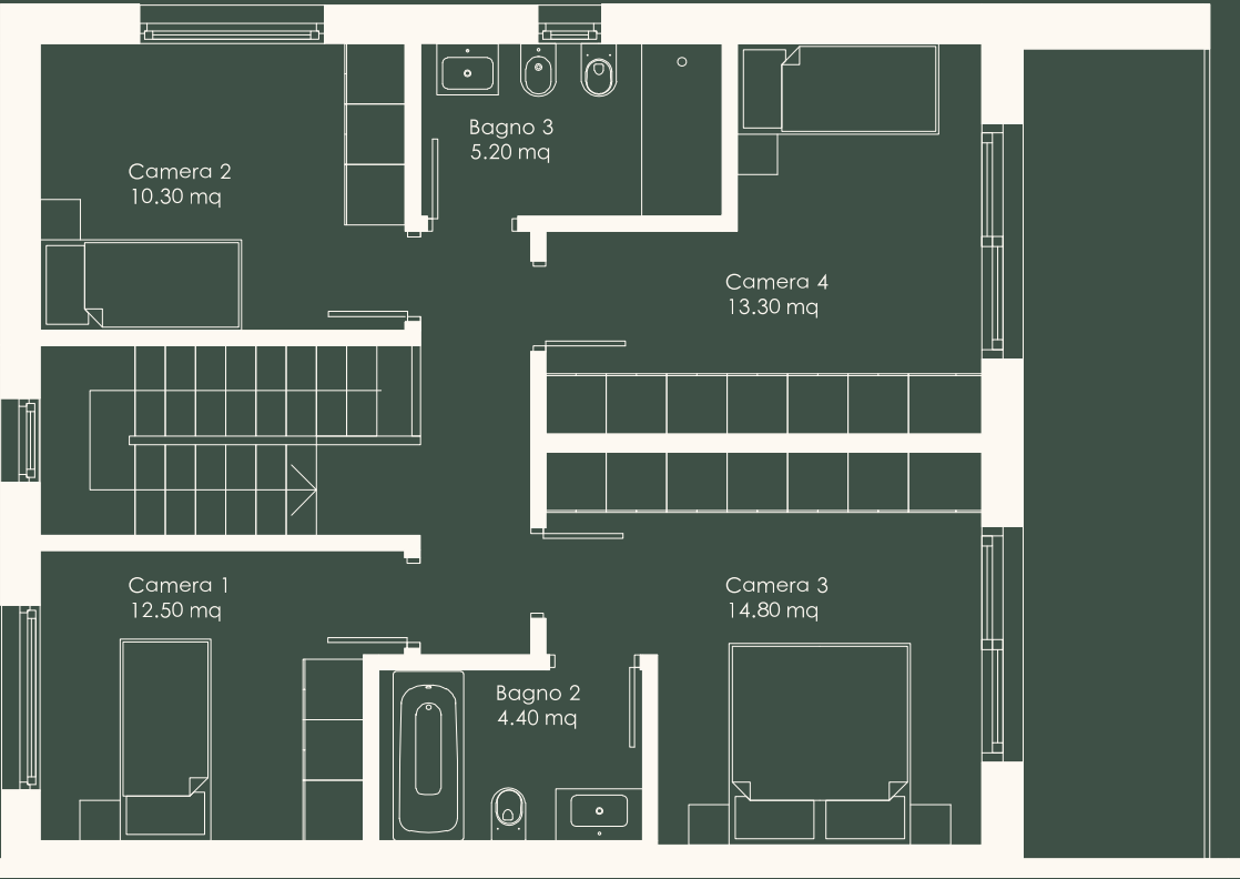
Primo Piano
