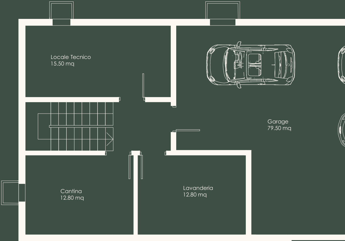
Primo interrato
