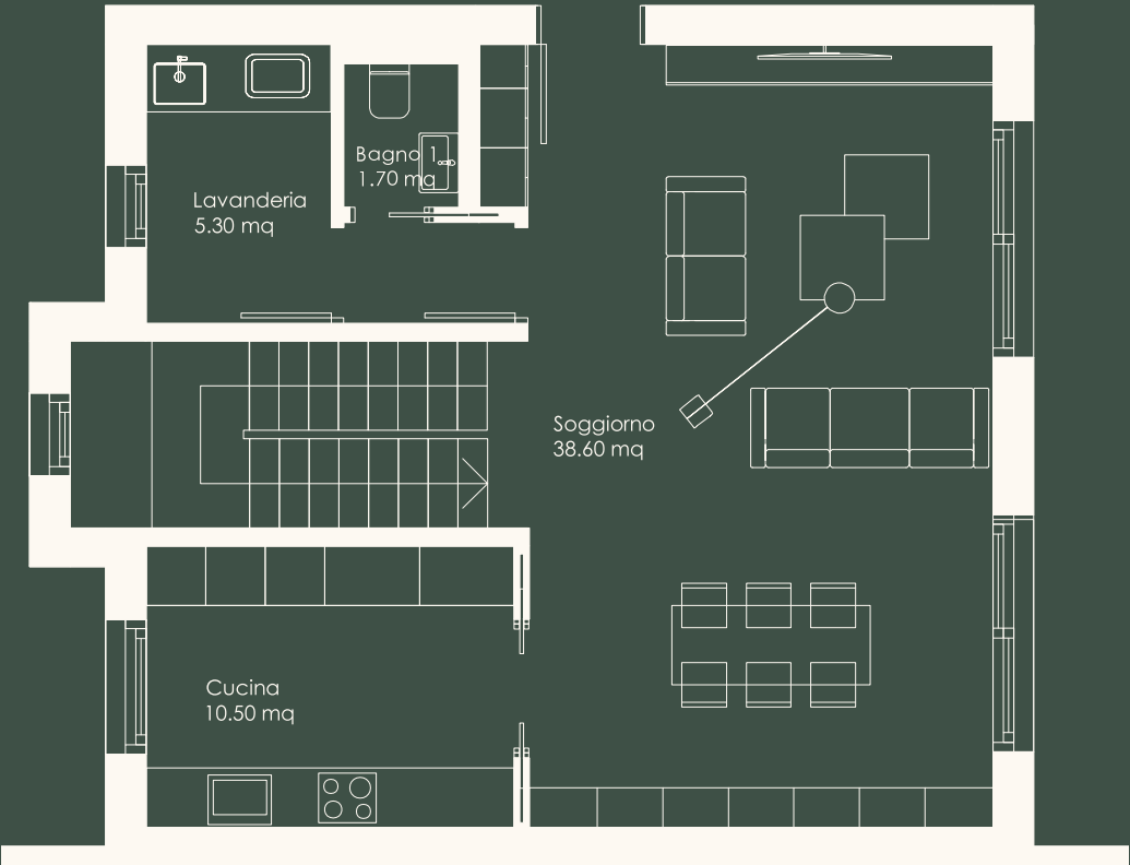
Primo Piano
