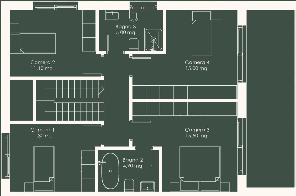
Primo Piano
