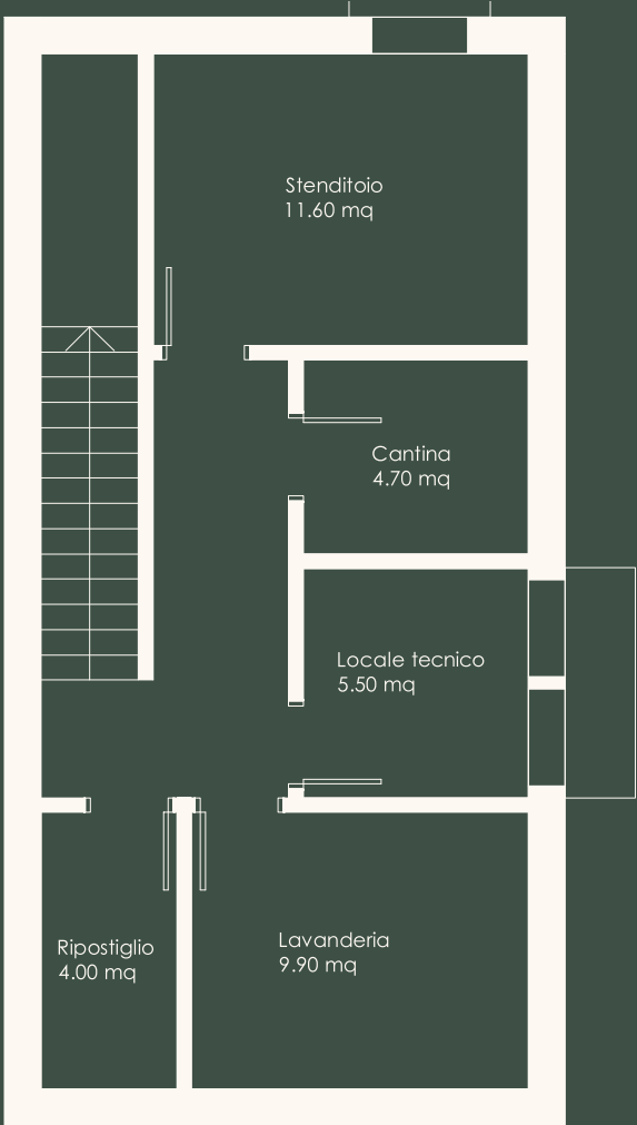
Primo interrato
